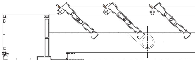
Coupe horizontale
