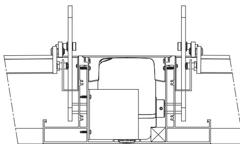
Coupe horizontale sans poteau central
