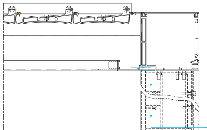
Coupe horizontale poteaux affleurants
