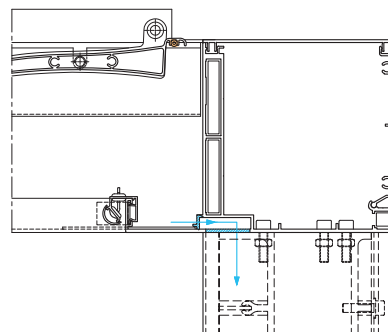
Coupe horizontale poteaux alignés + luminaire
