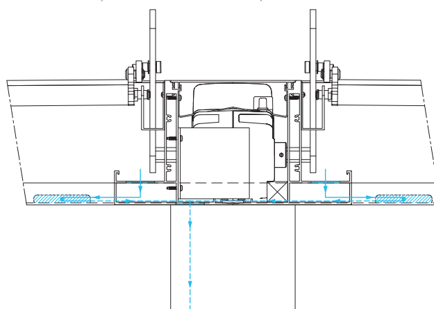
Coupe horizontale avec poteau central
